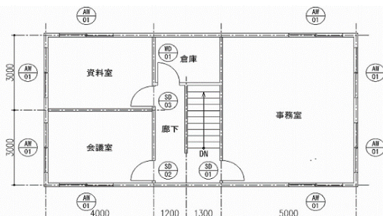
【建具図】
